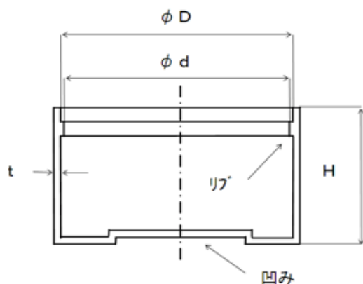
H型外径ネジ用 (パイプエンド) キャップ (管端部用 他)
