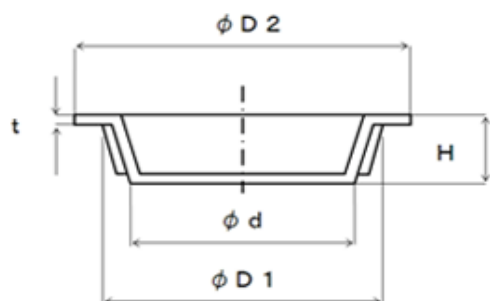
フランジ用 キャップ (鉄鋼製管フランジ用)
