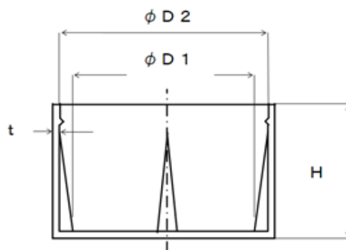
ソケット用 キャップ (鉄管溶接式フランジ用)
