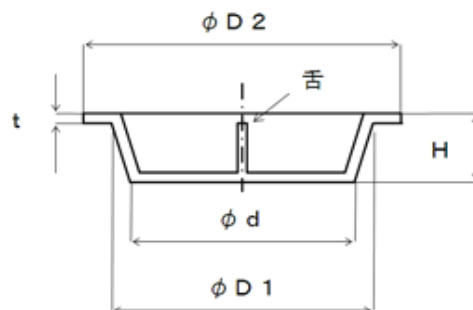
ネジ込み用 キャップ (管用メネジ用)
